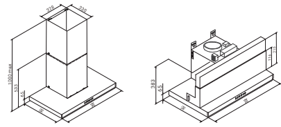
機體尺寸(含風管護罩) 機體尺寸(含伸縮護罩)
