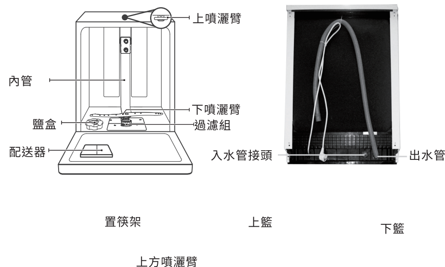
前視圖
