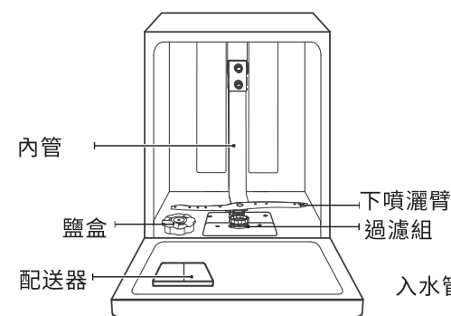
前視圖
