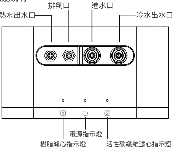
電子式觸控龍頭 D211×W55×H224mm
