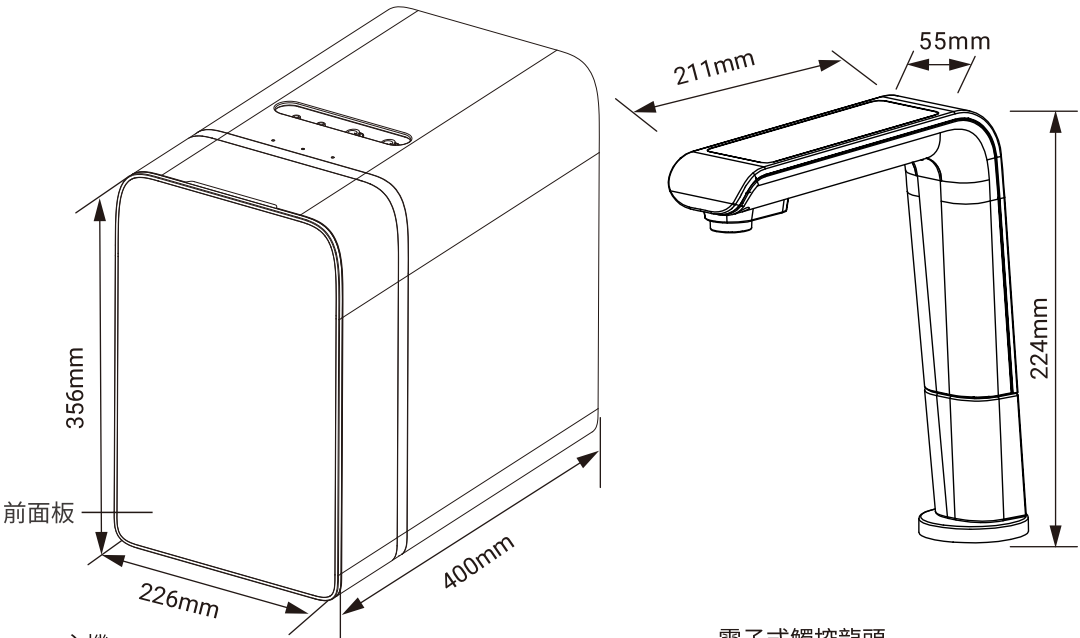
主機 D400×W226×H356mm
