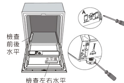
【圖6】腳調整圖示 註:腳的最大調整行程是50mm
